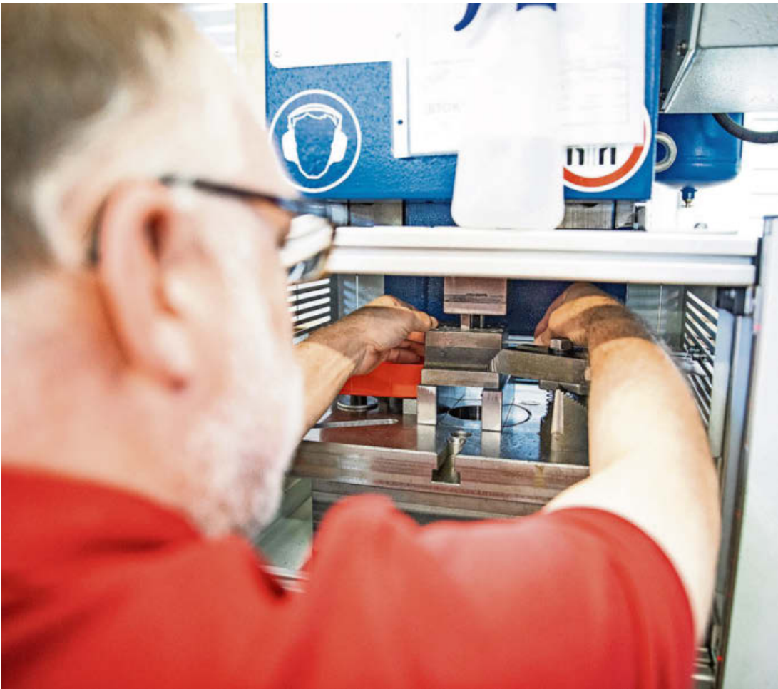
Ein grosser Teil der Lochplatten und Profile wird im Gehörlosendorf an einer Stanzmaschine hergestellt. Foto: PD
